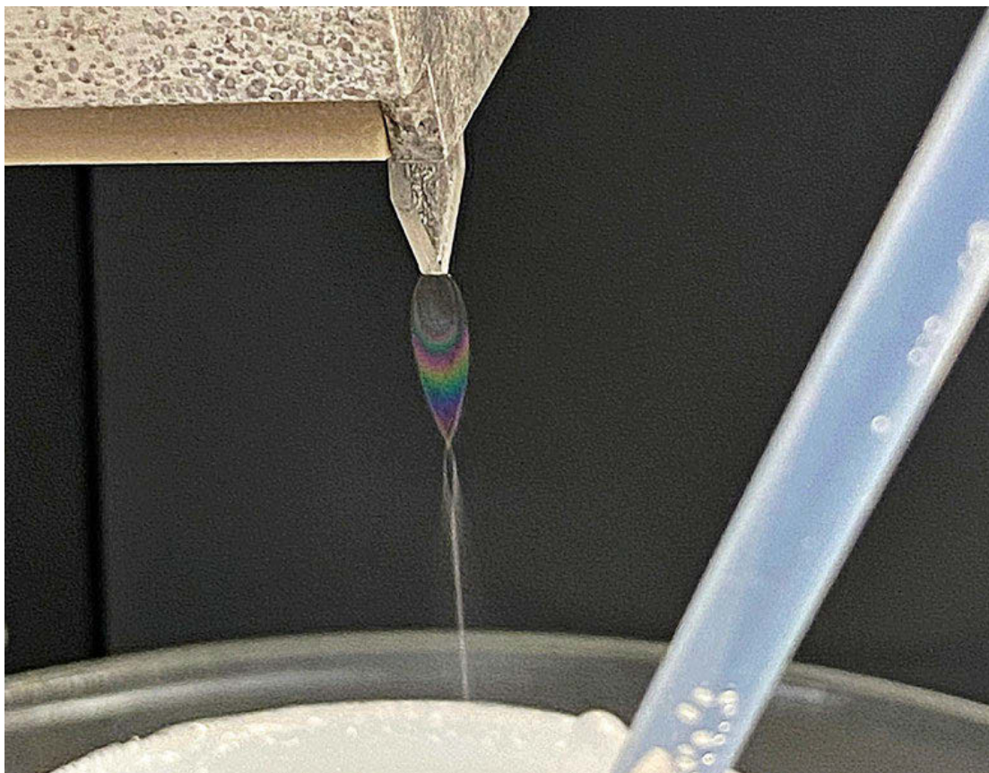
Lámina de agua líquida de un centímetro de ancho, seleccionada como objetivo del haz de rayos X. EMILY NIENHUIS
